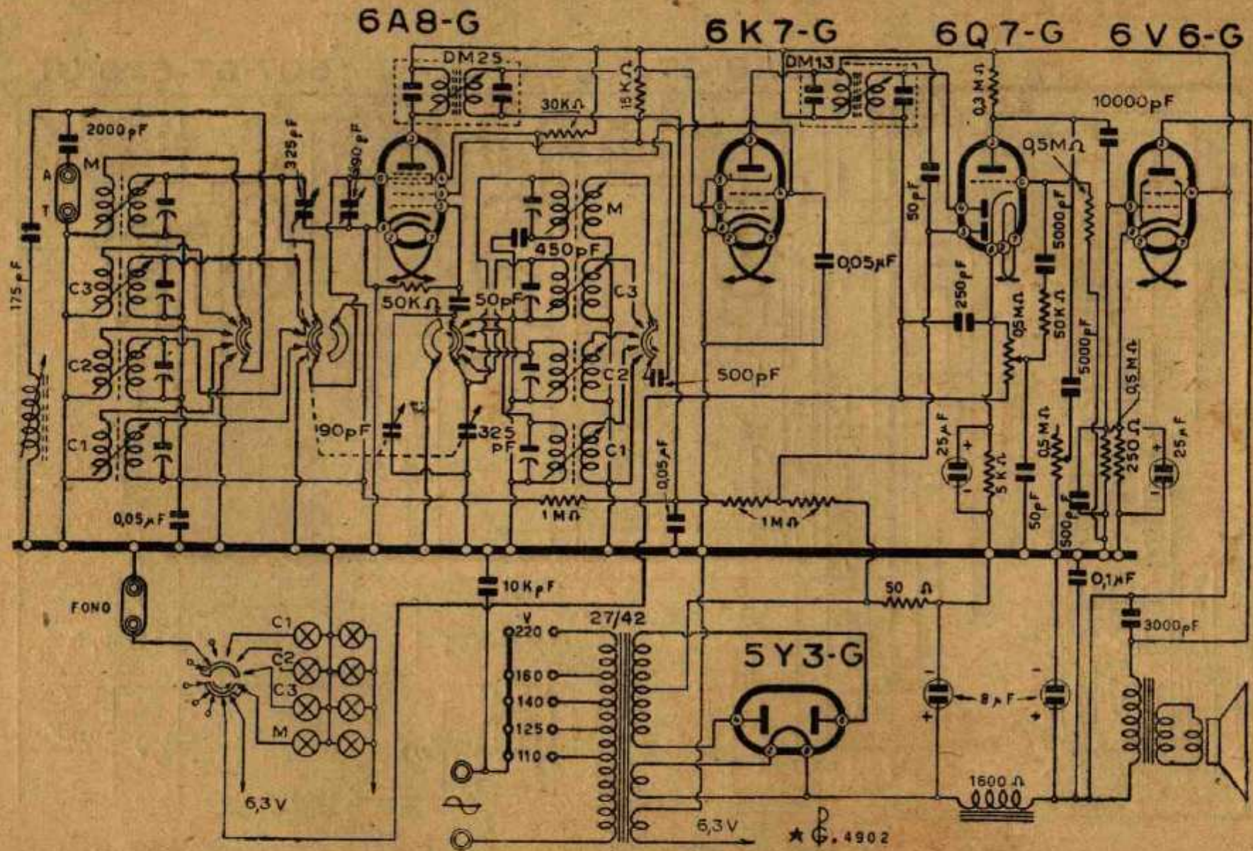
Lo schema elettrico del mod. 544 I. M. E. R. denominato "Verbano.. Il "Verbano II°" è lo stesso châssis montato come radiofonografo.
